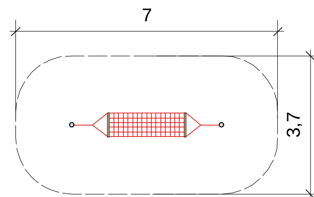
8 3 Stk. Hängematte an je 2 Stahlpfosten, farbig pulverbeschichtet
